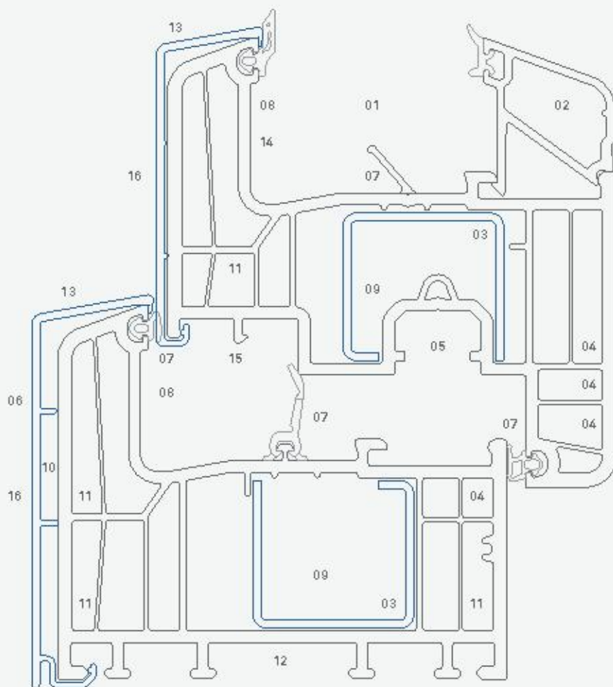
Eforte s hliníkovým krytom Obr.: 1:1
