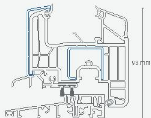
Novinka: Bezbariérový prah balkónových dverí Obr.: 1:2
